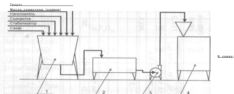
Рис. 14.1. Схема технологического процесса производства плавленного сыра: 1 — оборудование для термической обработки смеси (котел типа «Штефан»); 2 — емкость для промежуточного хранения смеси; 3 — насос для вязких продуктов; 4 — автомат для расфасовки в стаканчики
