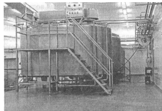
Рис. 8.1. Сыроизготовитель для производства сыра
