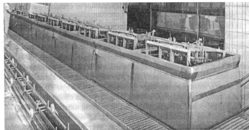
Рис. 9.2. Отделение посолки сыра в рассоле
