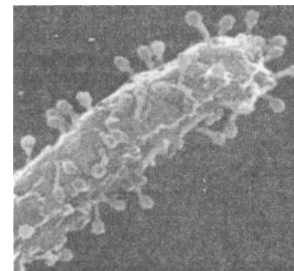
Рис- 6-4. Поражение клетки фагом
