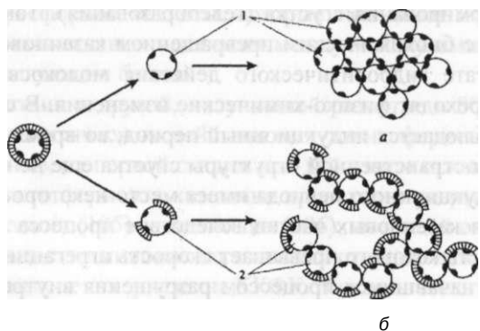
Рис. 7.2. Схематическое изображение истинной коагуляции и гелеобразования: а — истинная коагуляция; б — гелеобразование; 1 — частицы, полностью потерявшие фактор устойчивости; 2 — частицы, частично потерявшие фактор устойчивости
