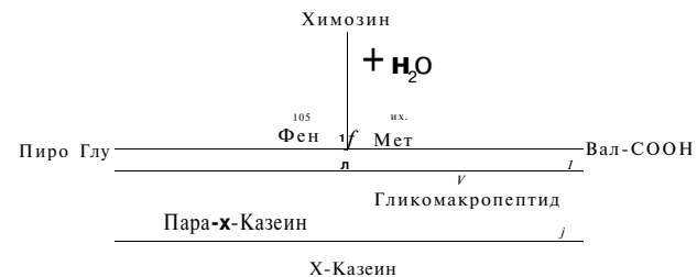
Рис. 7.1. Действие сычужного фермента на белки молока
