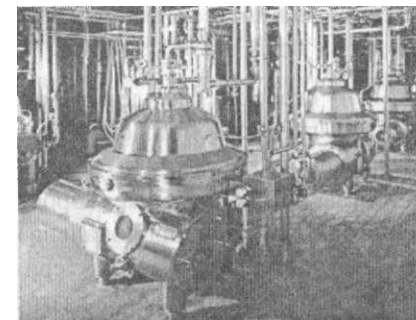
Рис. 4.1. Сепараторы
