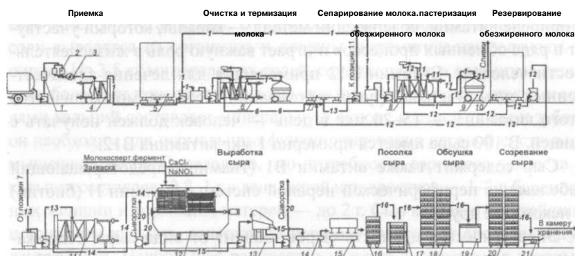
Рис. 2.2. Принципиально-конструктивная схема технологической линии производства сыра:
